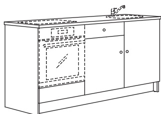
Kogumõõtmed: 182×61 cm
