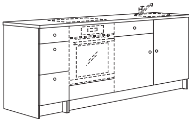
Kogumõõtmed: 244×61 cm
