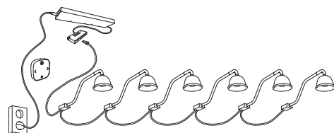
30 W TRÅDFRI draiveriga saad ühendada kuni 18 lampi, kuid need peavad olema jagatud maksimaalselt 6 lambiga gruppideks.
